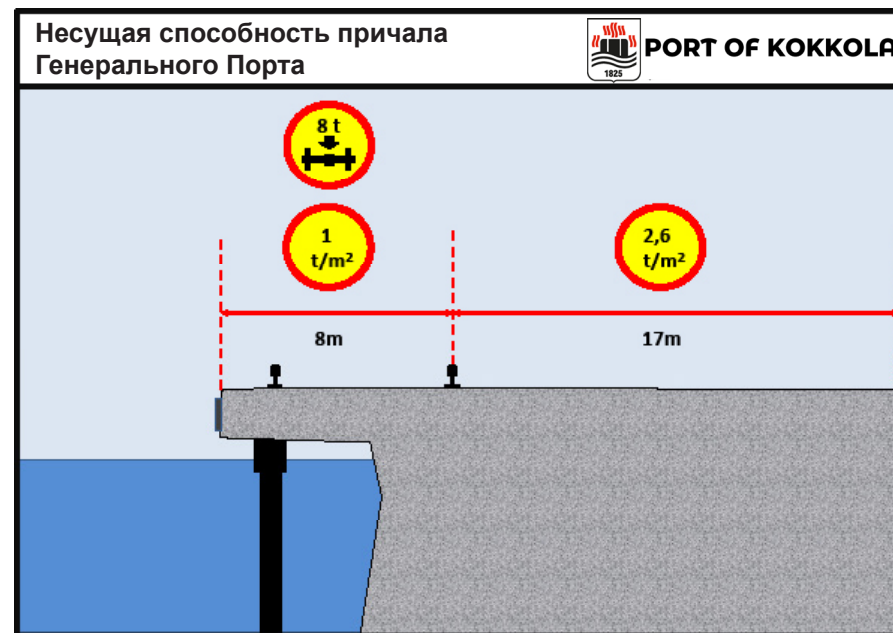
Несущая способность причала Генерального Порта
